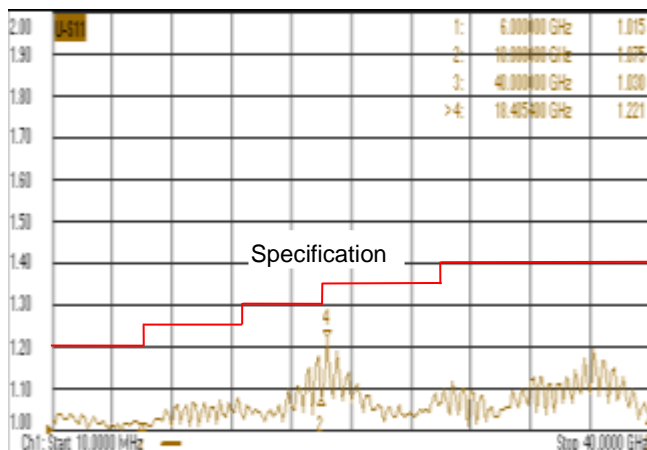
TC40-15-15-1000C 的典型 S11 指标:
