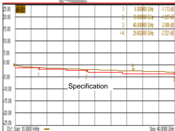
TC40-15-15-1000C 的典型 S21 指标:
