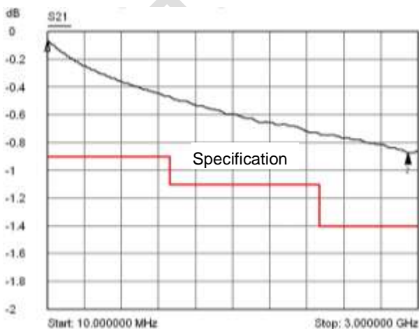
RD316-01-01-500 的典型 S21 指标:
