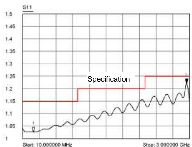
RD316-01-01-500 的典型 S11 指标:
